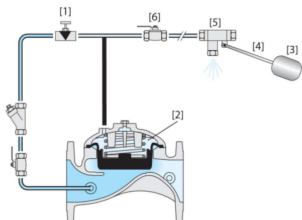
Válvula Aberta
