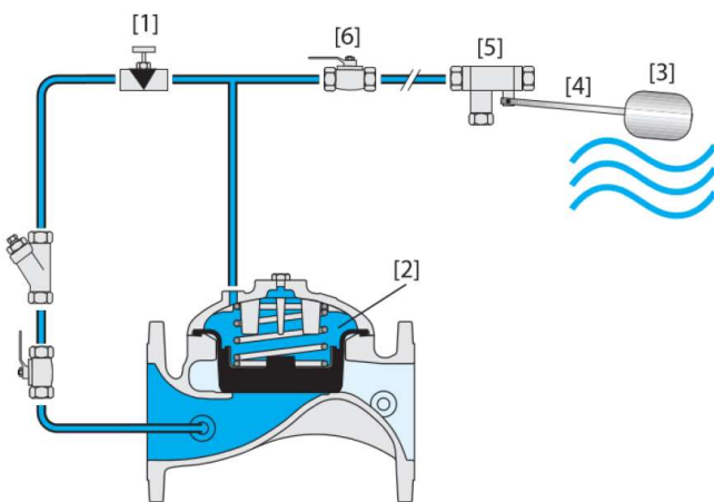
Válvula Fechada
